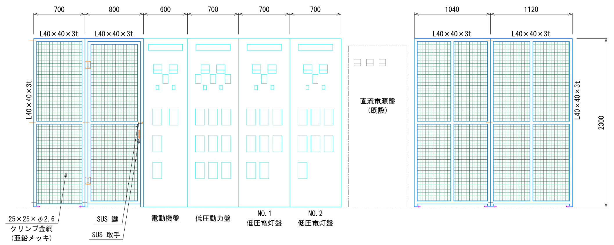
C-C 矢 視 図
