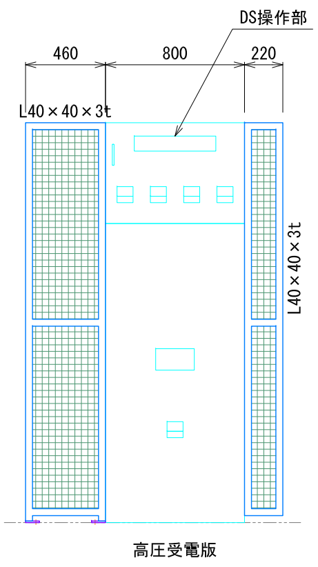
B-B 矢 視 図
