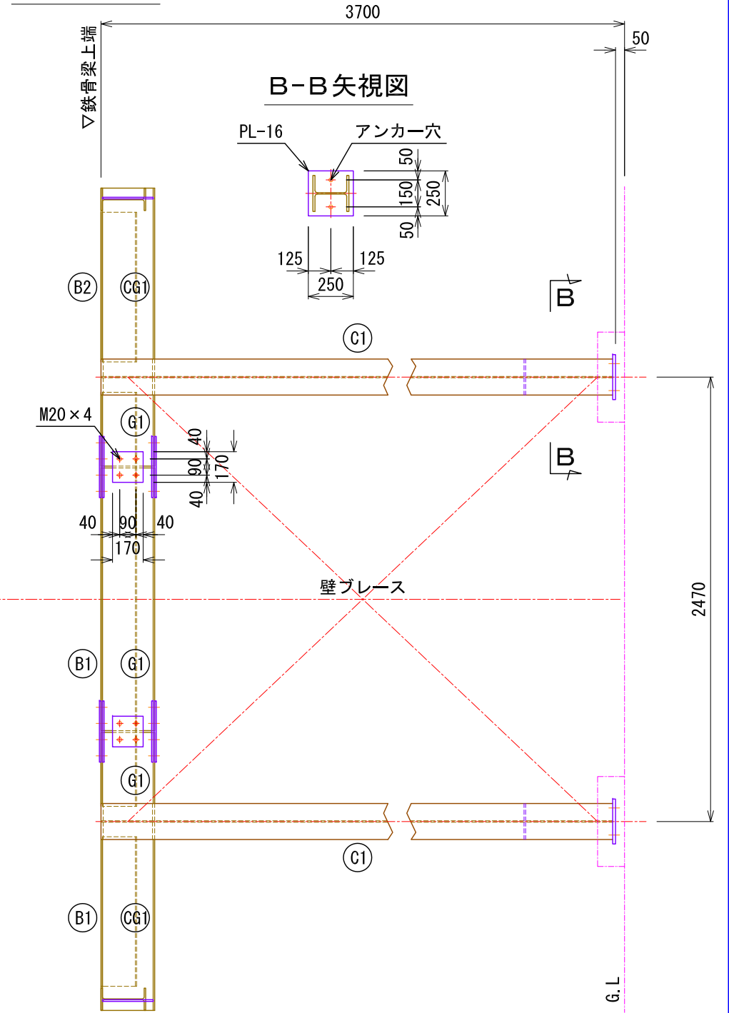
鉄骨側面図
