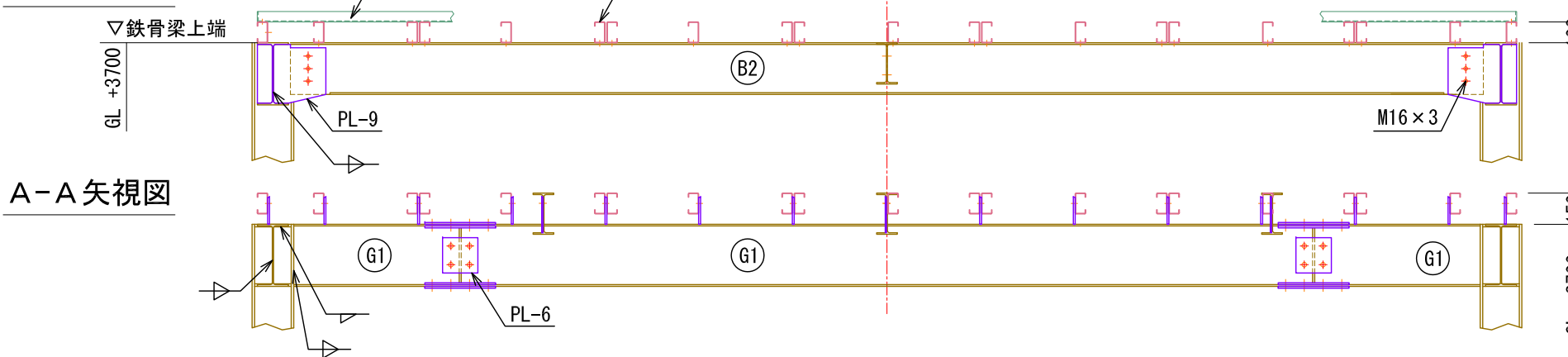
鉄骨正面図
