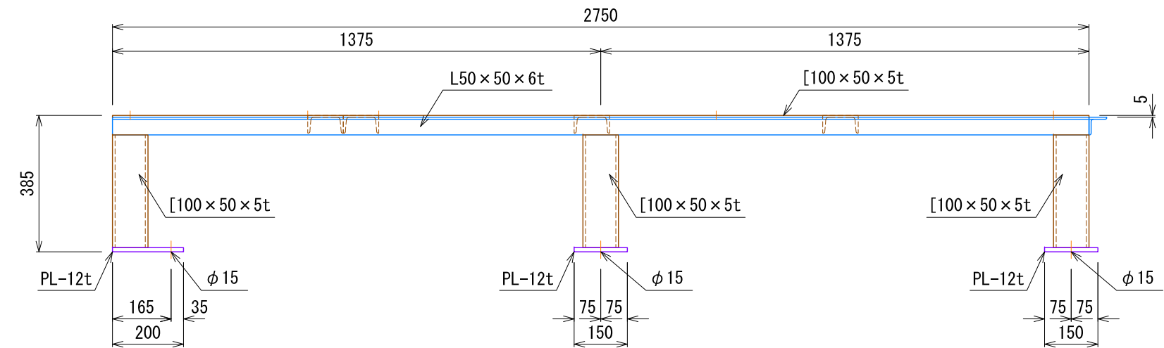
正面図
