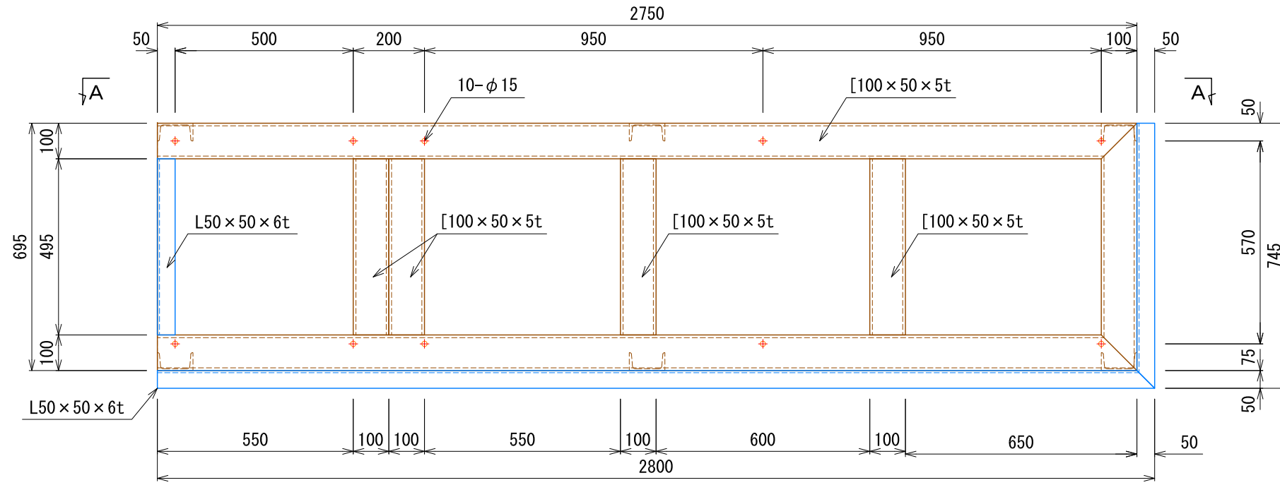
上面図
