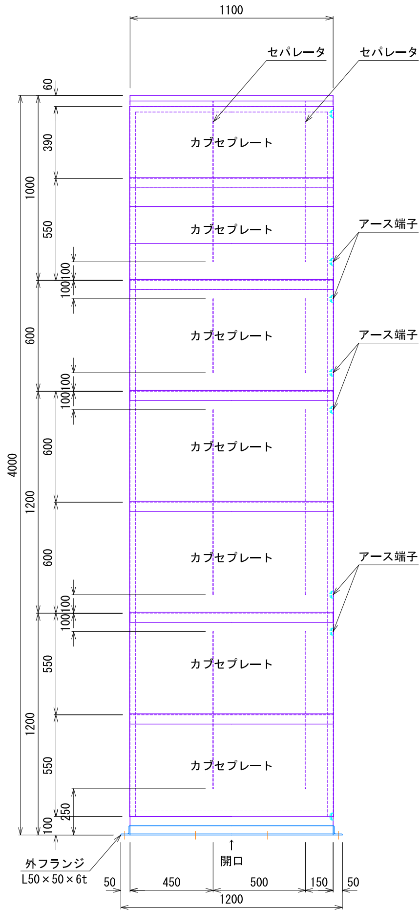
正面図
