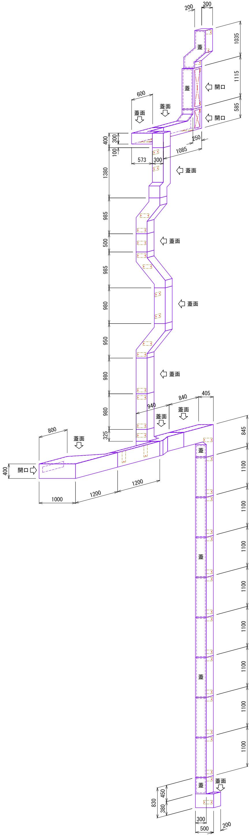
ワイヤリングダクト ①
